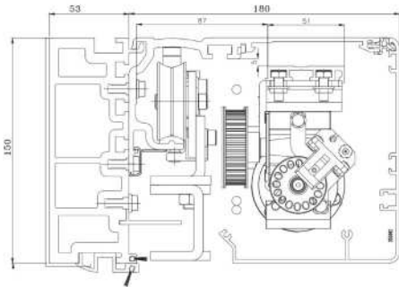
KABA - SLM
