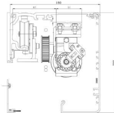
DORMA - ES200
